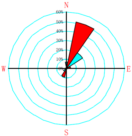
风能玫瑰图
