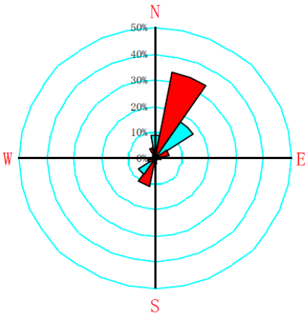
风向玫瑰图
