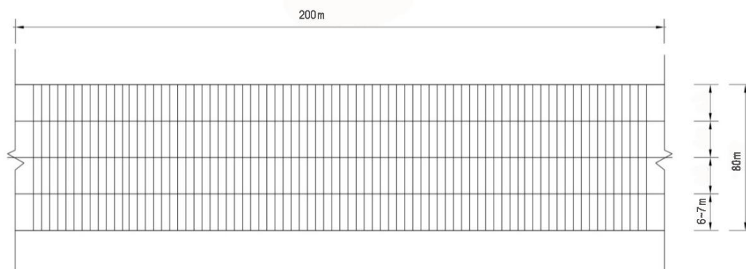
图 1.6-2 养殖筏基本单元平面图
