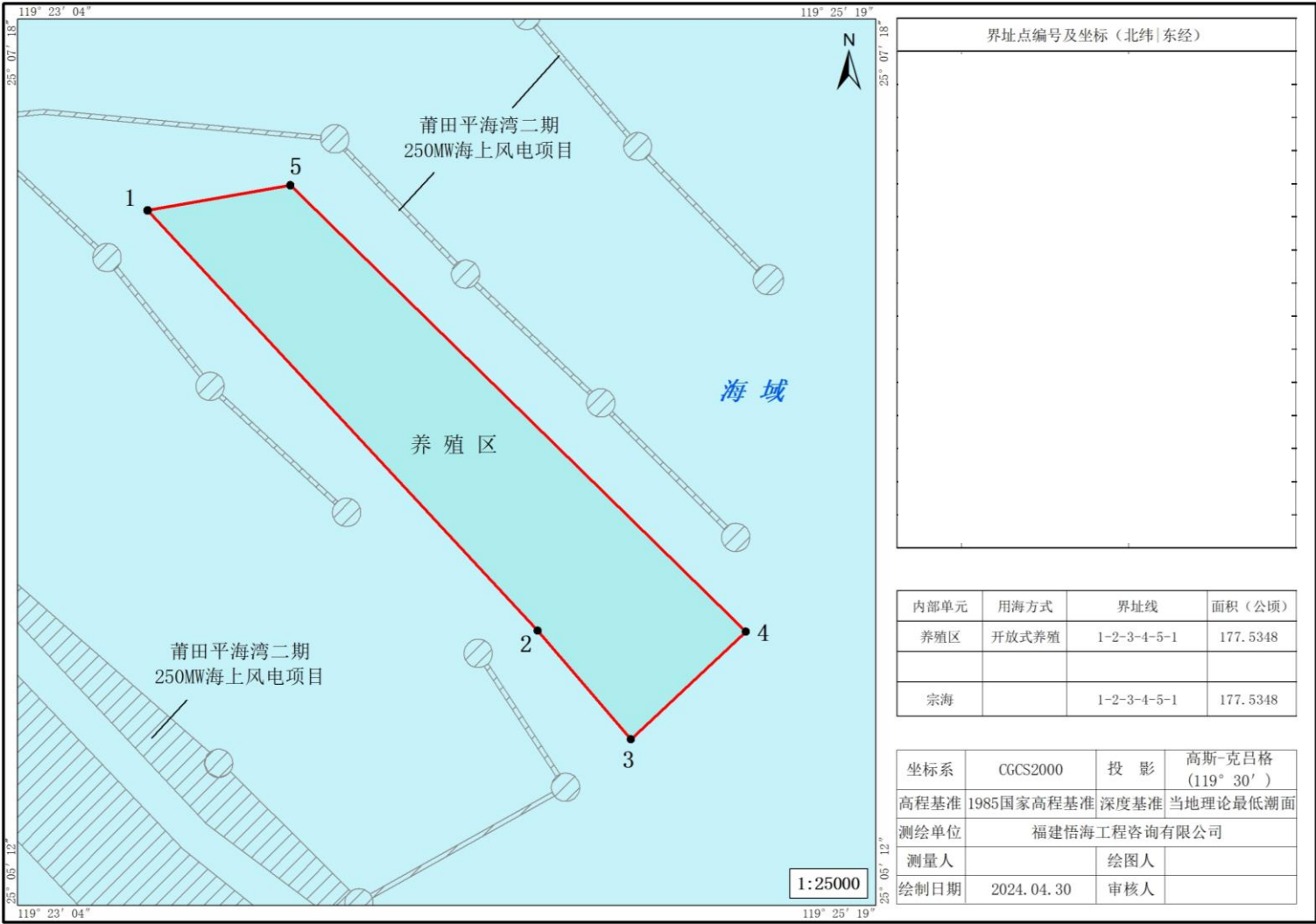
莆田平海湾海上风电场三期开放式养殖区块（三）项目宗海界址图
