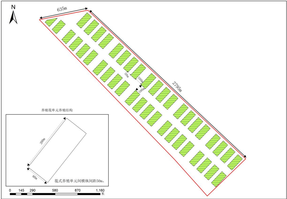
图 1.3-1 总平面布置示意图
