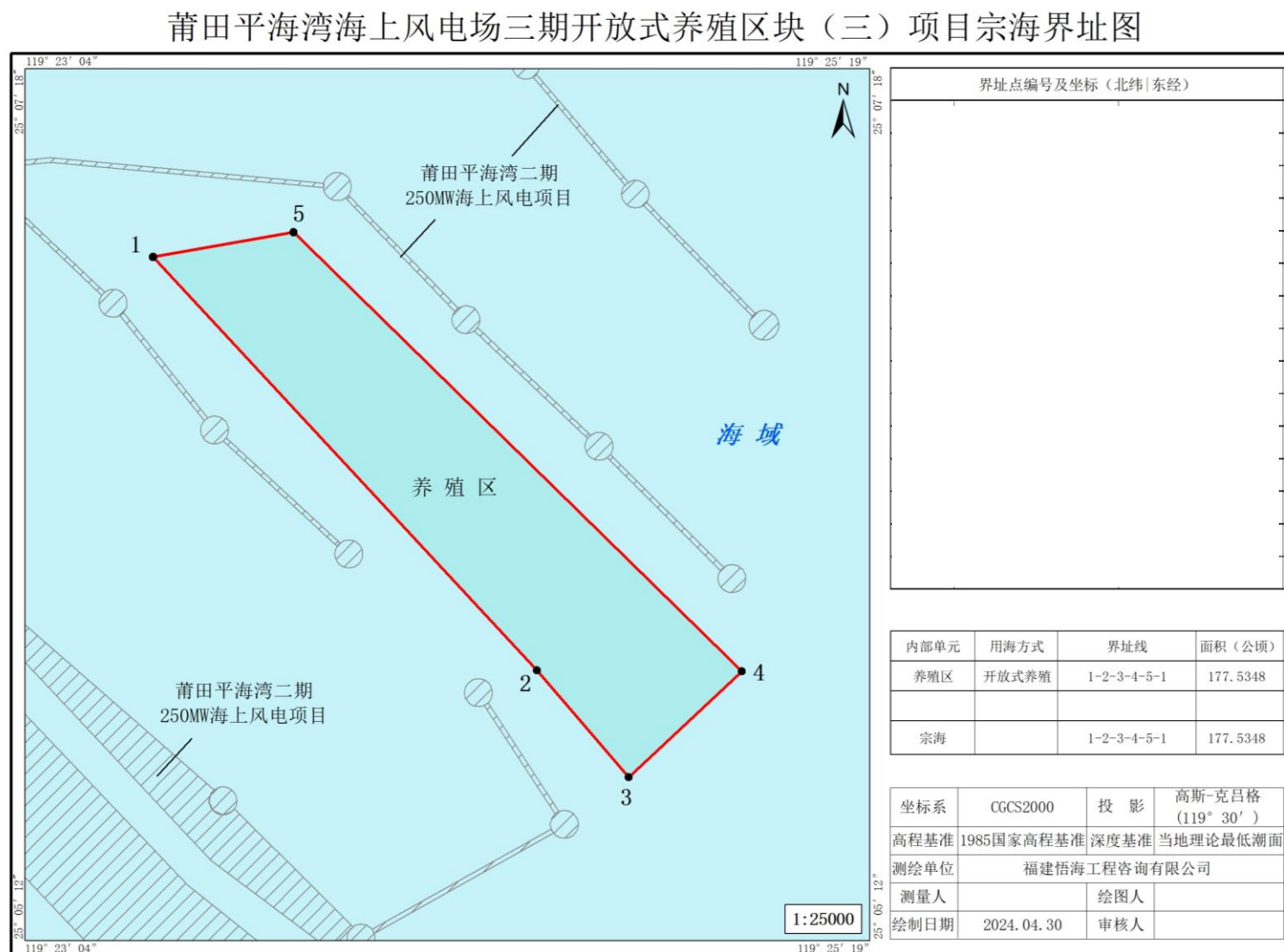
图 1.5-2 项目宗海界址图
