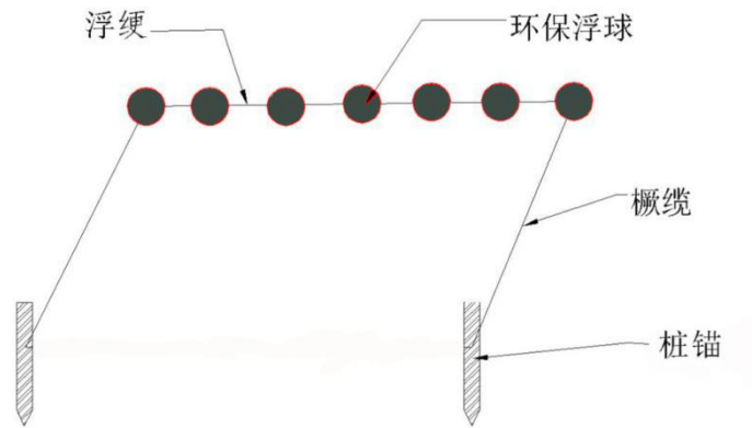
图 1.3-3 养殖筏断面图
