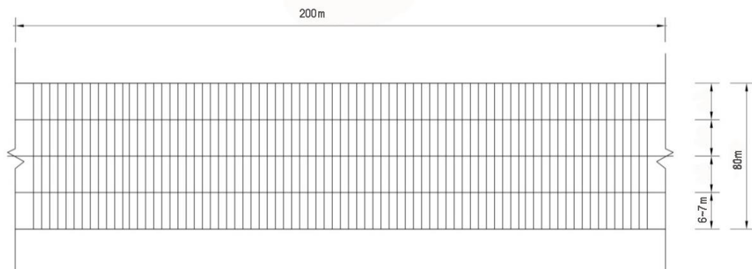
图 1.3-2 养殖筏基本单元平面图
